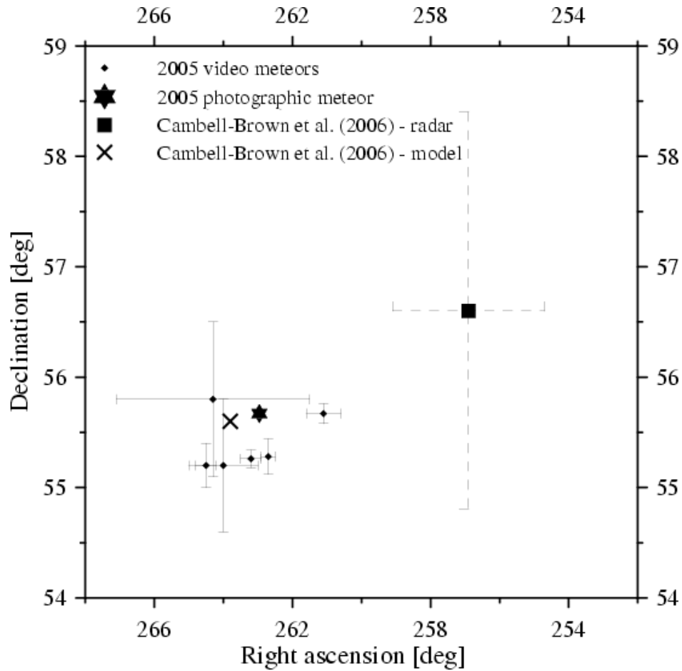
Εικόνα 3.4 Ακτινοβόλα σημεία των Δρακοντίδων της έξαρσης του 2005 από διαφορετικές τεχνικές. Οι κάθετες και οριζόντιες γραμμές αντιπροσωπεύουν τα σφάλματα μέτρησης. Πηγή: Koten et al, A&A, 466, 729-735, 2007.
