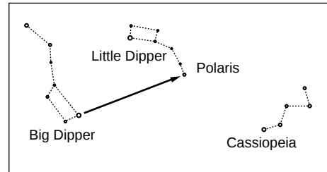
Fig. 26: Locating Polaris.
